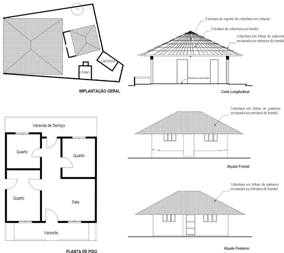
Figura 5. Casa em Paquitequete (fonte: desenho dos autores com base em Carrilho (2005))
