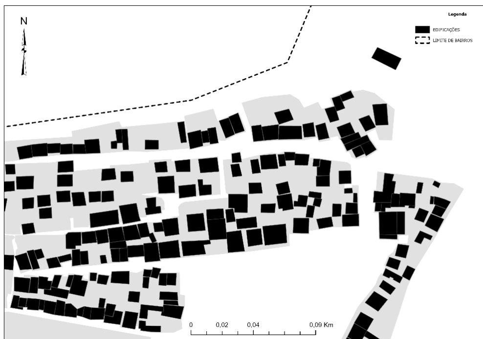
Figura 10. Cheios e vazios distinguindo limite da praia, casas e lotes (talhões) (fonte: desenho de Iracema Carlos Andrade com base em mapas do Portal WebGIS de Moçambique)
